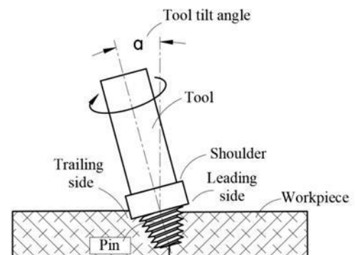
Fig. 5 Tool tilt angle
