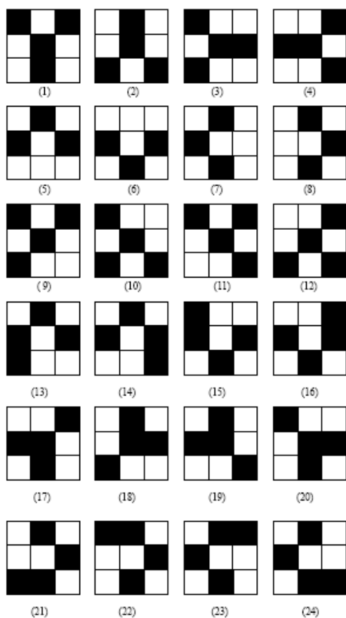
Fig. 4 Bifurcation Templates
